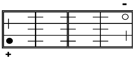
Schaltung 24 Volt DIN C
