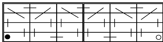
Schaltung 48 Volt DIN C
