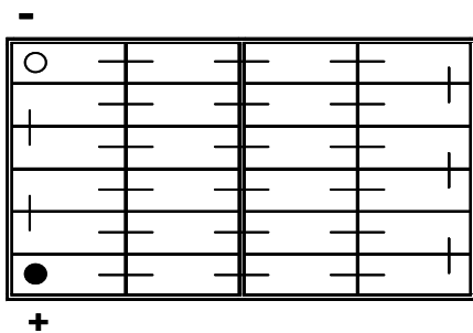
Schaltung 48 Volt DIN A
