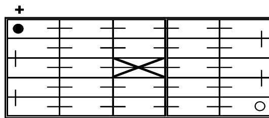
Schaltung 48 Volt DIN C
